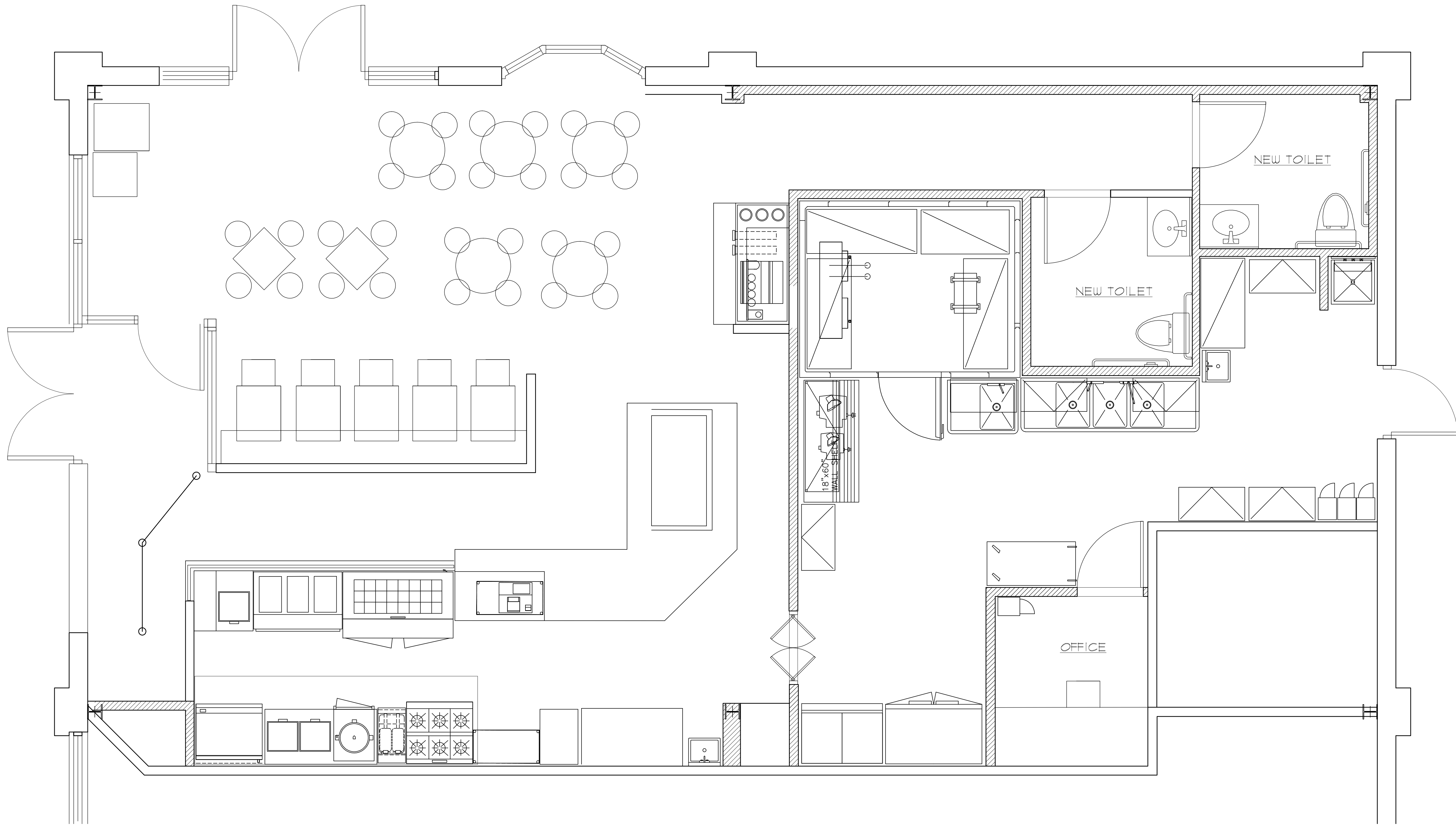
1 FLOOR PLAN A-1 SCALE: 1/8" = 1'-0"
